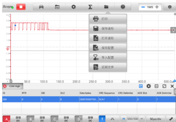
图 9-28 “文件菜单”界面示意图
