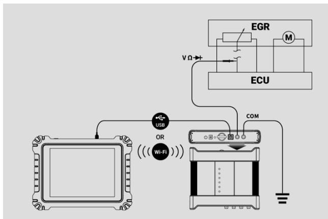
图 9-92 直流电压连接示意图
