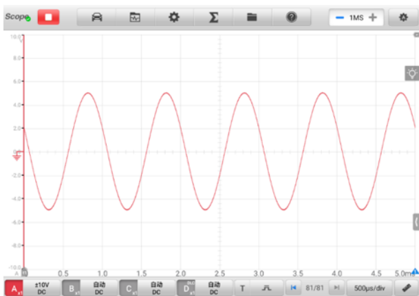
图 9-32 “通道选择” 界面示图 2 (未选择)
