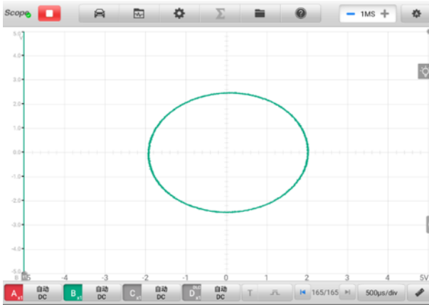
图 9-13 “XY 视图” 界面示意图
