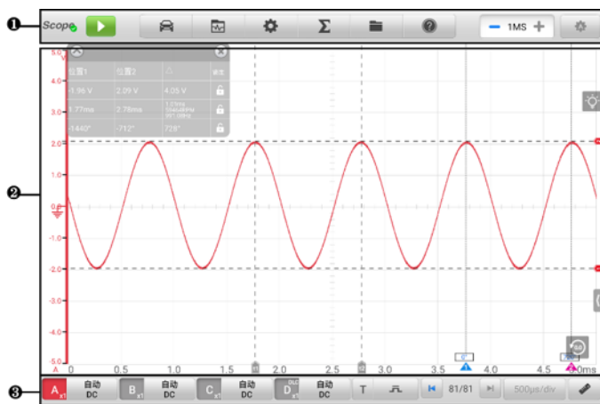
图 9-4 “示波器主页”示意图
