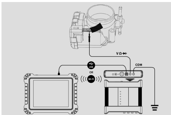
图 9-62 万用表连接示意图
