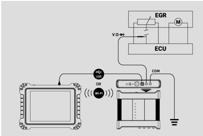
图 9-83 信号发生器连接图示图
