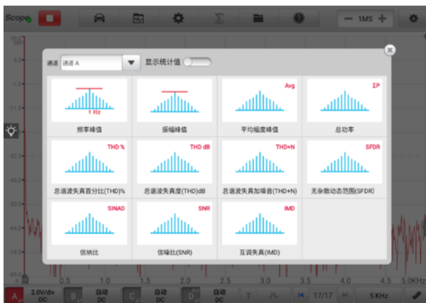
图 9-59 测量示图 (频谱视图)
