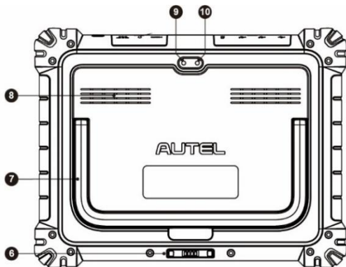
图 2-2 MaxiSys 平板诊断设备后视图
