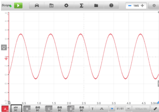
图 9-42 “幅值设置”界面示意图 2 (AC 5 V)
