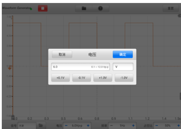
图 9-99 电压设置示意图 2
