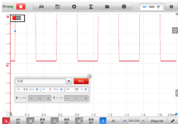
图 9-30 “超量程”界面示图
