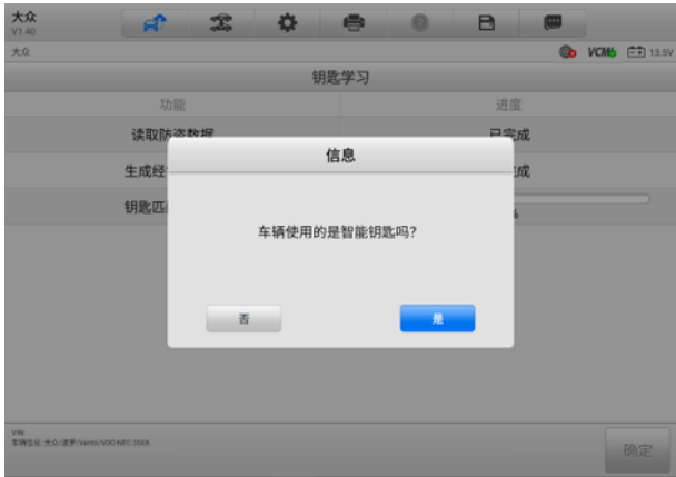
图 8-9 “钥匙学习” 界面示意图 4
