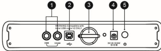
图 2-5 MaxiFlash VCMII 顶视图
